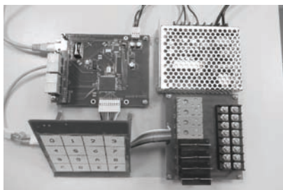
本校自行研發設計之電化設備監控裝置硬體電路板
